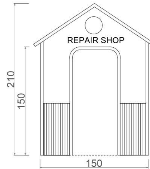
ÖN GÖRÜNÜŞ
